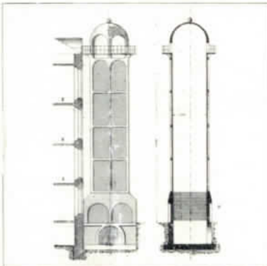
Выполнено для Т-на Зуевской М-ры (башня) ст. Дрезна. Московск. губ.
