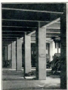
Выполнено для Г. г. Бр. Анатра (железобетонные перекрытия мельницы) в Одессе.
