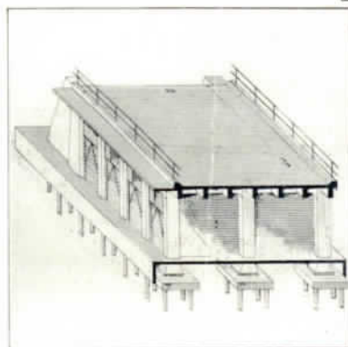
Выполнено для Г-на А. А. Злотницкого (железобетонная мостовая со шпалой) Ружинь, Киевск. губ.
